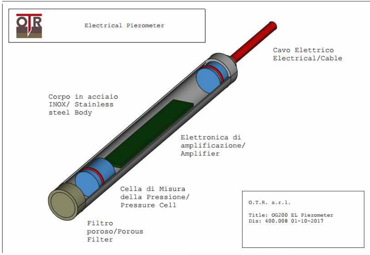
Figura 2 Piezometro Elettrico, Componenti
