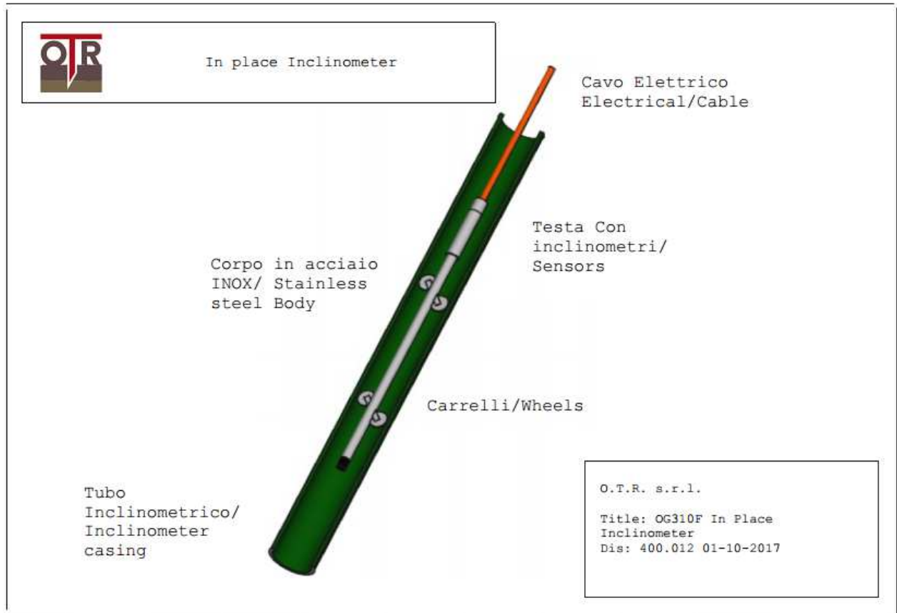
Figura 2 Parti sonda inclinometrica fissa
