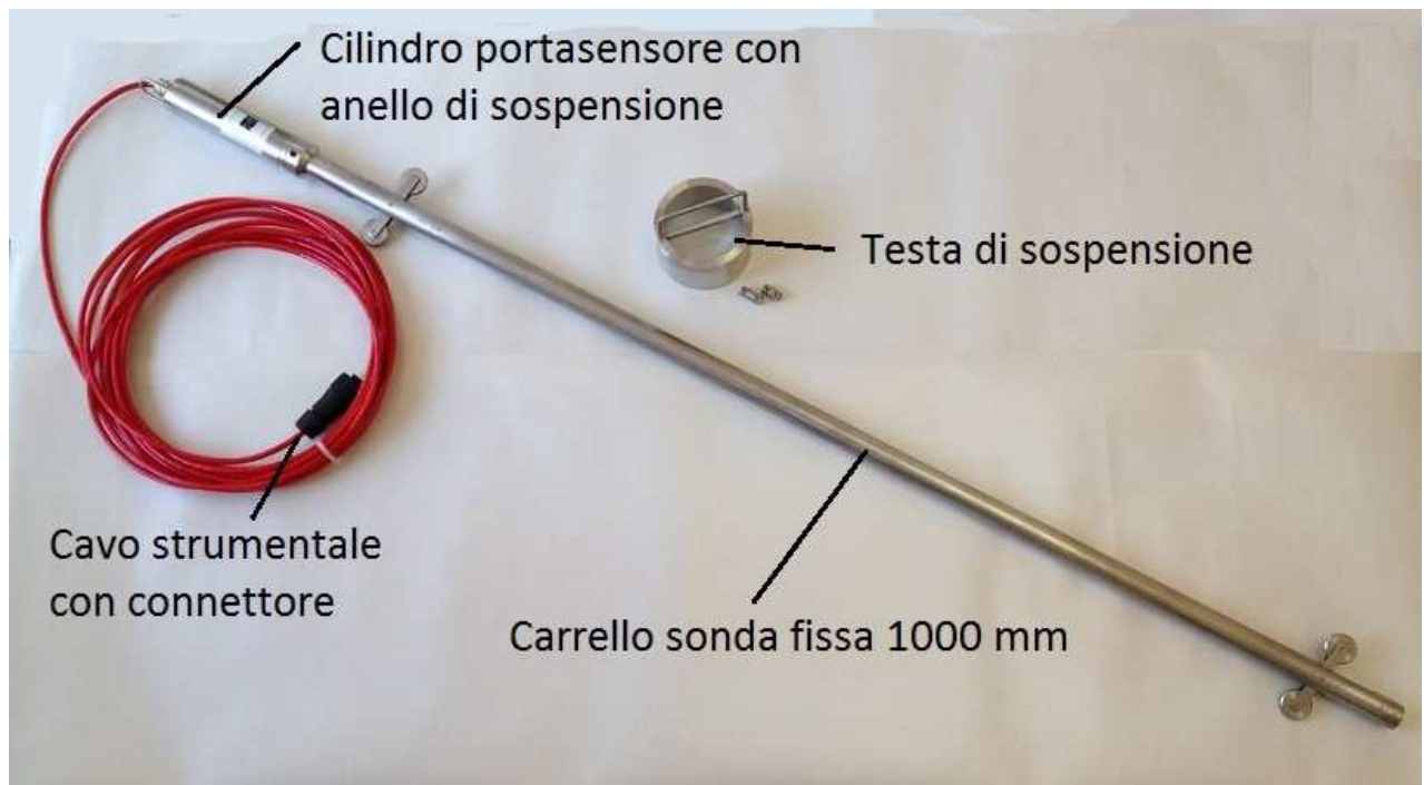
Fig. 1 – Sonda inclinometrica fissa di profondità
